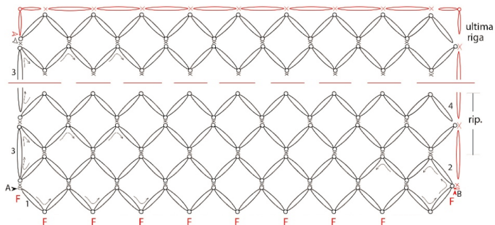
Schema 1: lavorazione a punto strega
